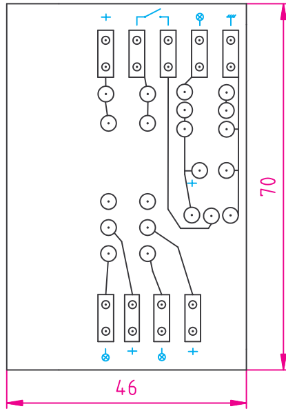
Strana mědi
