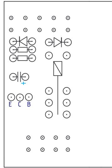
Osazení součástek
