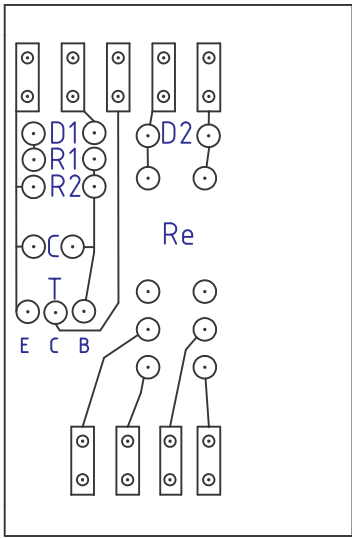
Strana součástek
